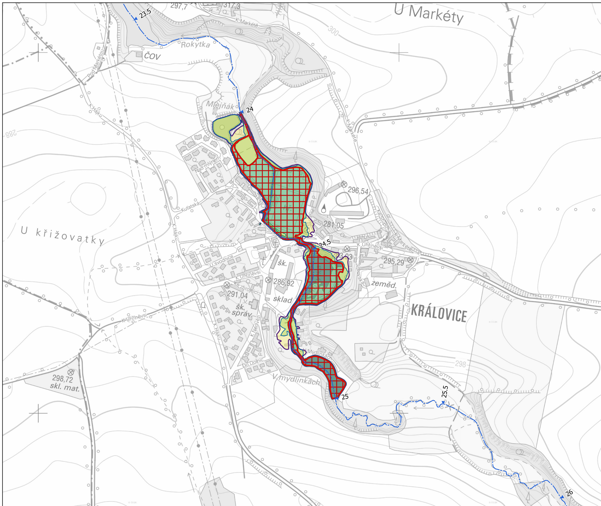
9. Mapa záplavových čar, záplavového území a aktivní zóny
